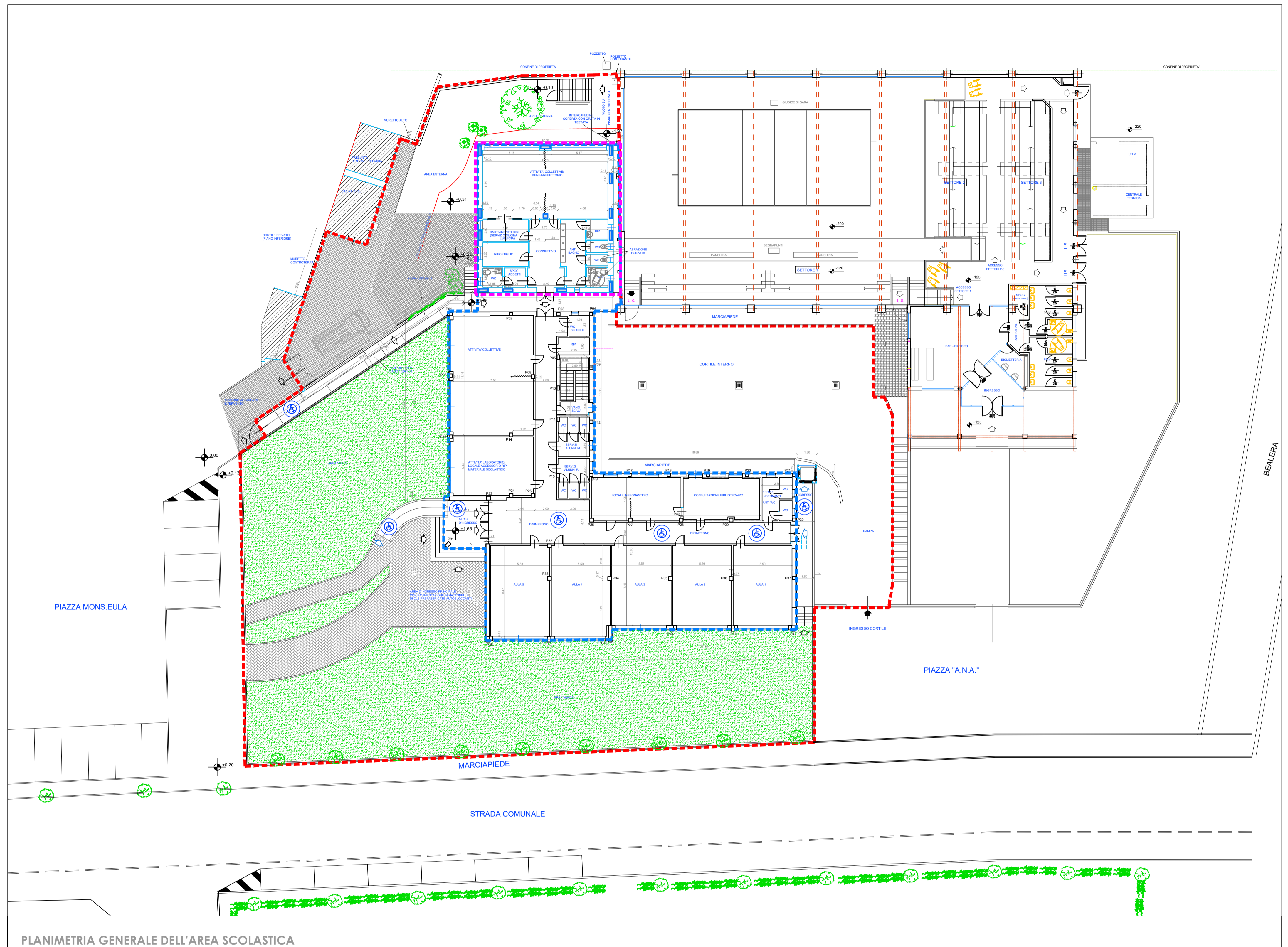
PLANIMETRIA GENERALE DELL'AREA SCOLASTICA
